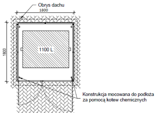
Boks Eko 1 Lite - rzut z góry
