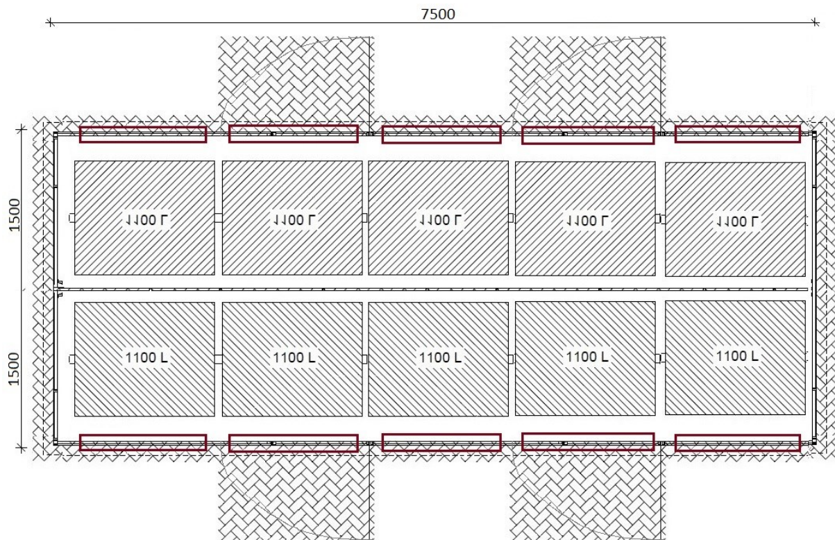
poglądowy rysunek techniczny rzut poziomy
