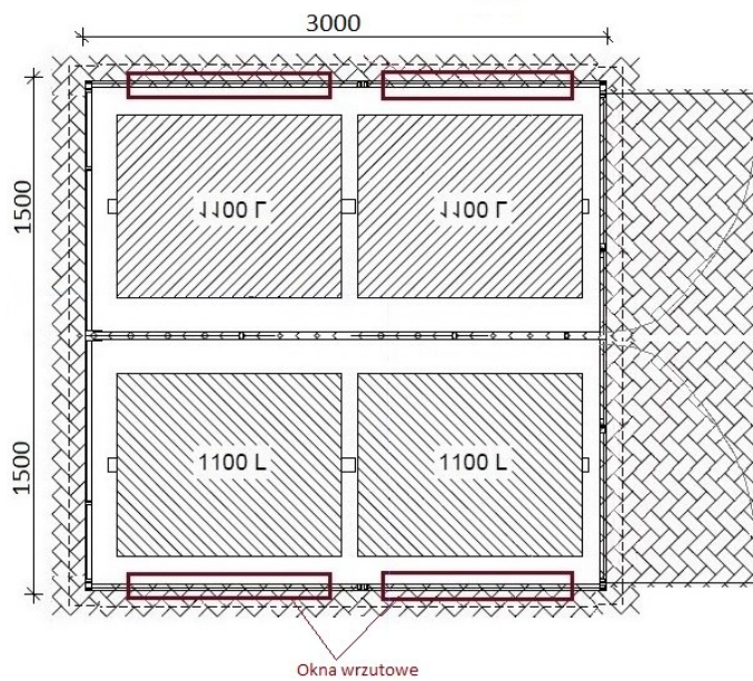
poglądowy rysunek techniczny rzut poziomy
