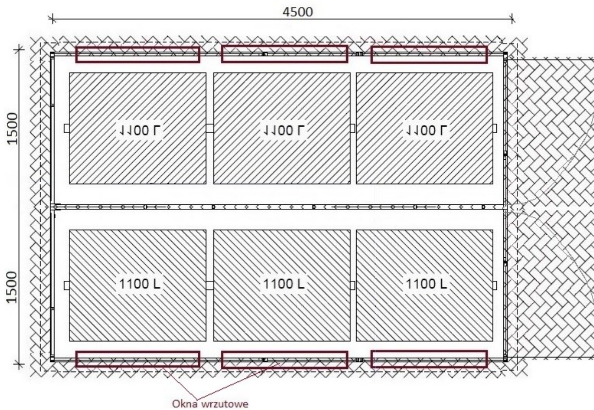
poglądowy rysunek techniczny rzut poziomy
