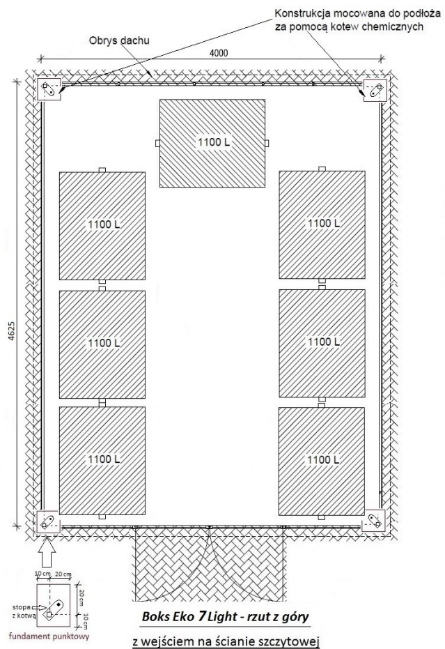
poglądowy rysunek techniczny rzut poziomy
