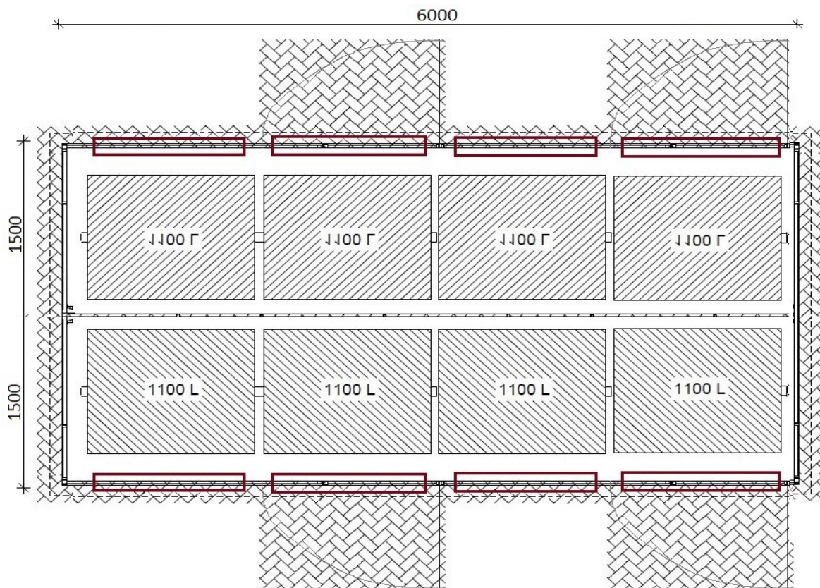
poglądowy rysunek techniczny rzut poziomy
